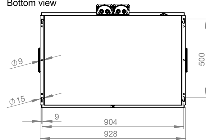
Ansicht von unten/ Bottom view
