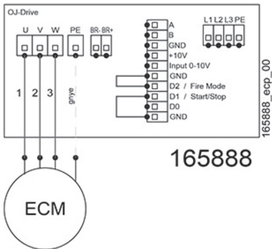
Aansluiting 0-10 V signaal
