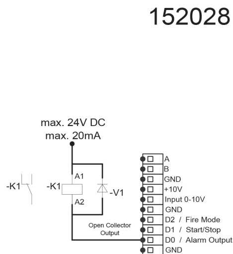
Relais met alarmuitgang geschakeld
