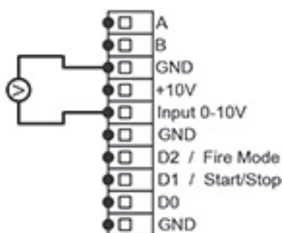
Aansluiting 0-10 V signaal
