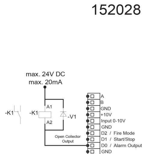
Relais met alarmuitgang geschakeld
